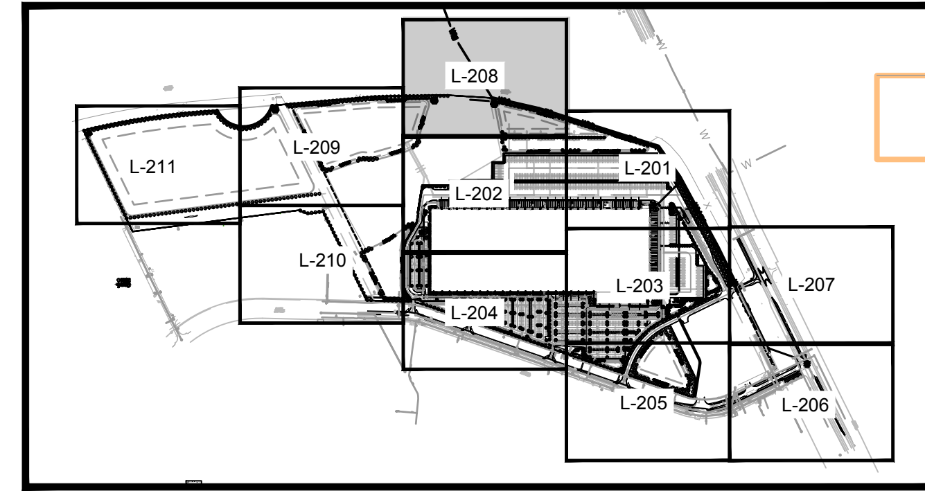
KEY MAP
