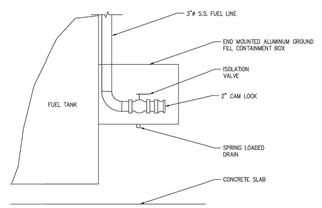
CONTAINMENT BOX DETAIL N.T.S.
